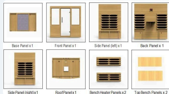
Componenti principali della cabina SmartSauna F4.
